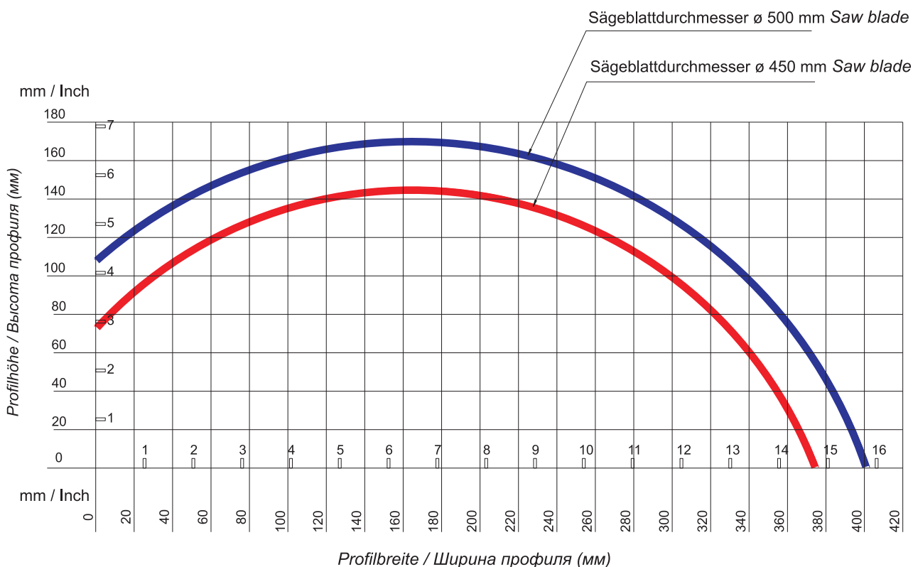
Abbildung 2: Schnittdiagramm UTK 90.
